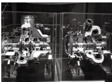
液体水素(左)と液体酸素(右) のターボポンプ
