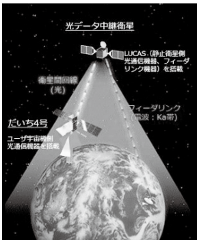
図は光データ中継システムの概要。「だいち4号」で取得された画像データが光データ中継衛星を経由して地上局に伝送される。
